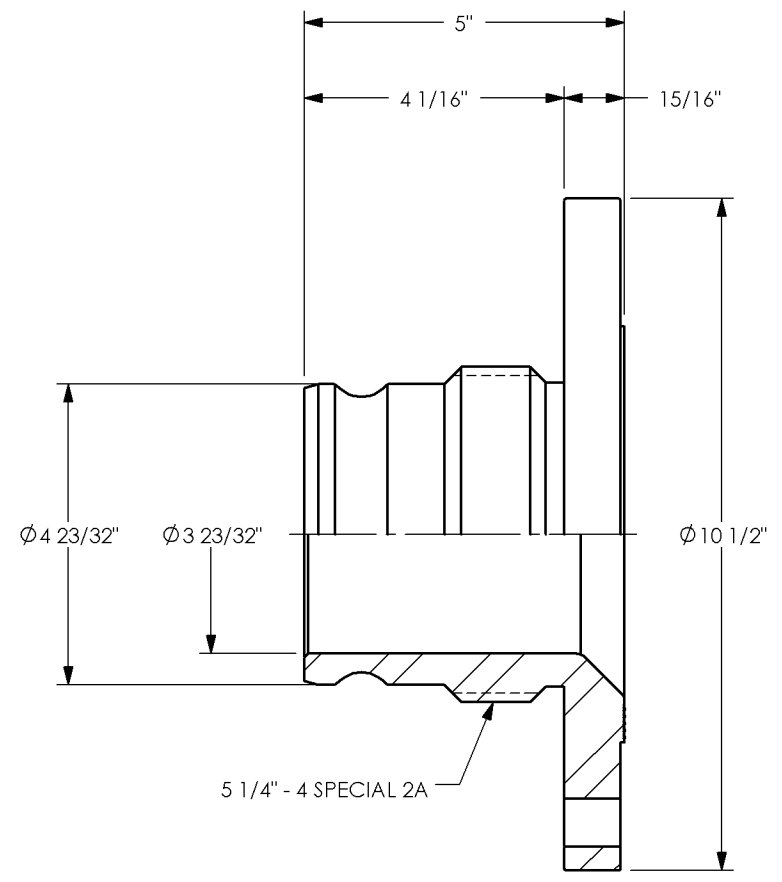
SECTION A-A
